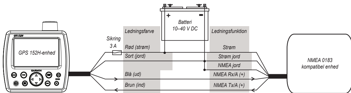
Tilslutning af en GPS 152H-enhed til en NMEA 0183-standardenhed
